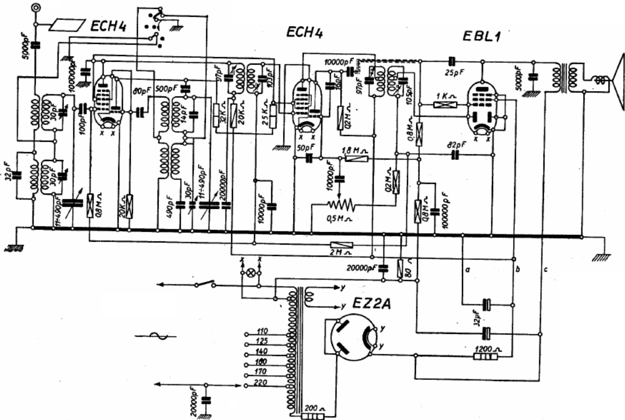
PHILIPS RADIO - Mod. BI 390 A e mod. BI 390 A bis - Onde corte e medie - Media frequenza 468 kc/s. Potenza d'uscita 2 W circa. Il mod. BI 390 A bis differisce per avere il condensatore elettrolitico 2 \times 50 \mu\text{F} . (V. modifica a parte).
